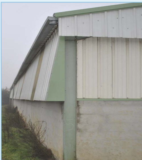
Solution initiale de ventilation latérale par bandeau translucide décalé
