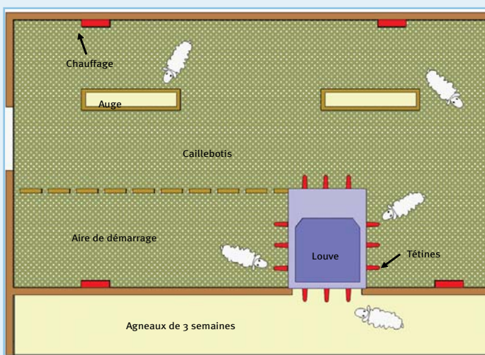
Figure 9 : Un exemple d'aménagement pour l'allaitement artificiel des agneaux
