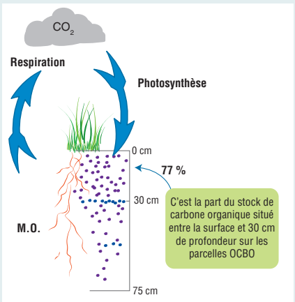
FIGURE 3 : LE CARBONE, UN CYCLE NATUREL ENTRE ATMOSPHÈRE, VÉGÉTAUX ET SOL
