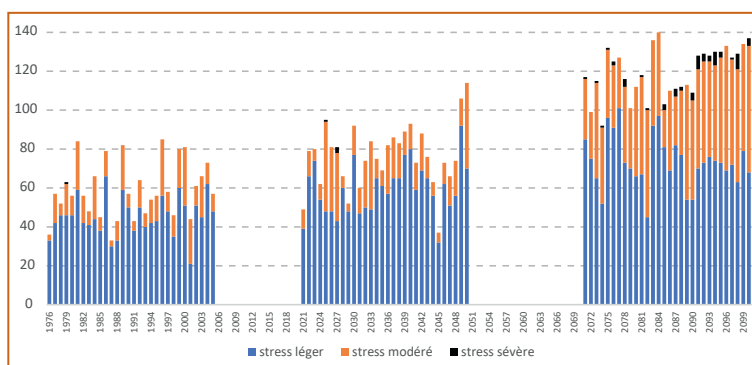
Figure 2 : Nombre de jours de stress des animaux à Sainte-Maure-de-Touraine (37)
