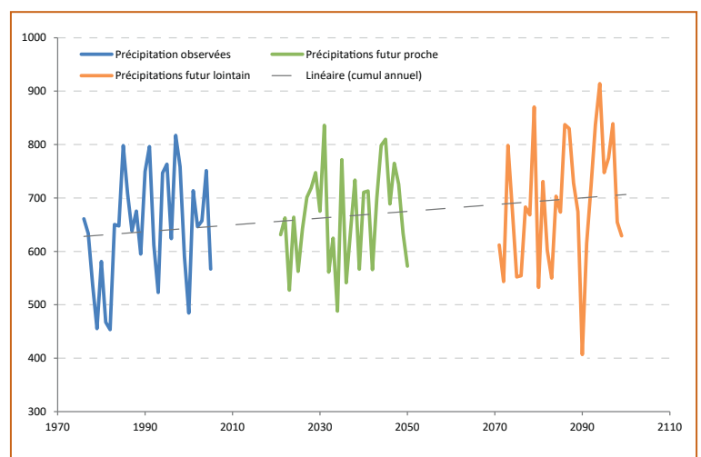
Figure 3 : Cumuls annuels de précipitations observés de 1986 à 2014, et prévus dans le futur à Sainte-Maure-de-Touraine (37)
