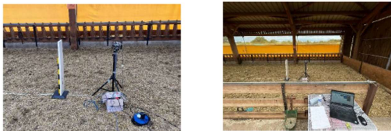
Test de l'antenne en condition d'élevage de brebis de différents stades physiologiques
